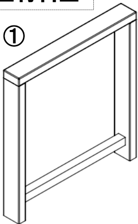
脚(600×80×650)・・・2本
