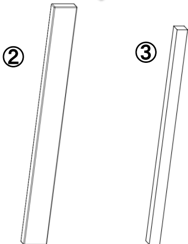
木材(900×85×35)・・・7本 木材(685×35×35)・・・1本
